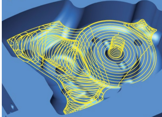
HPC 荒加工
